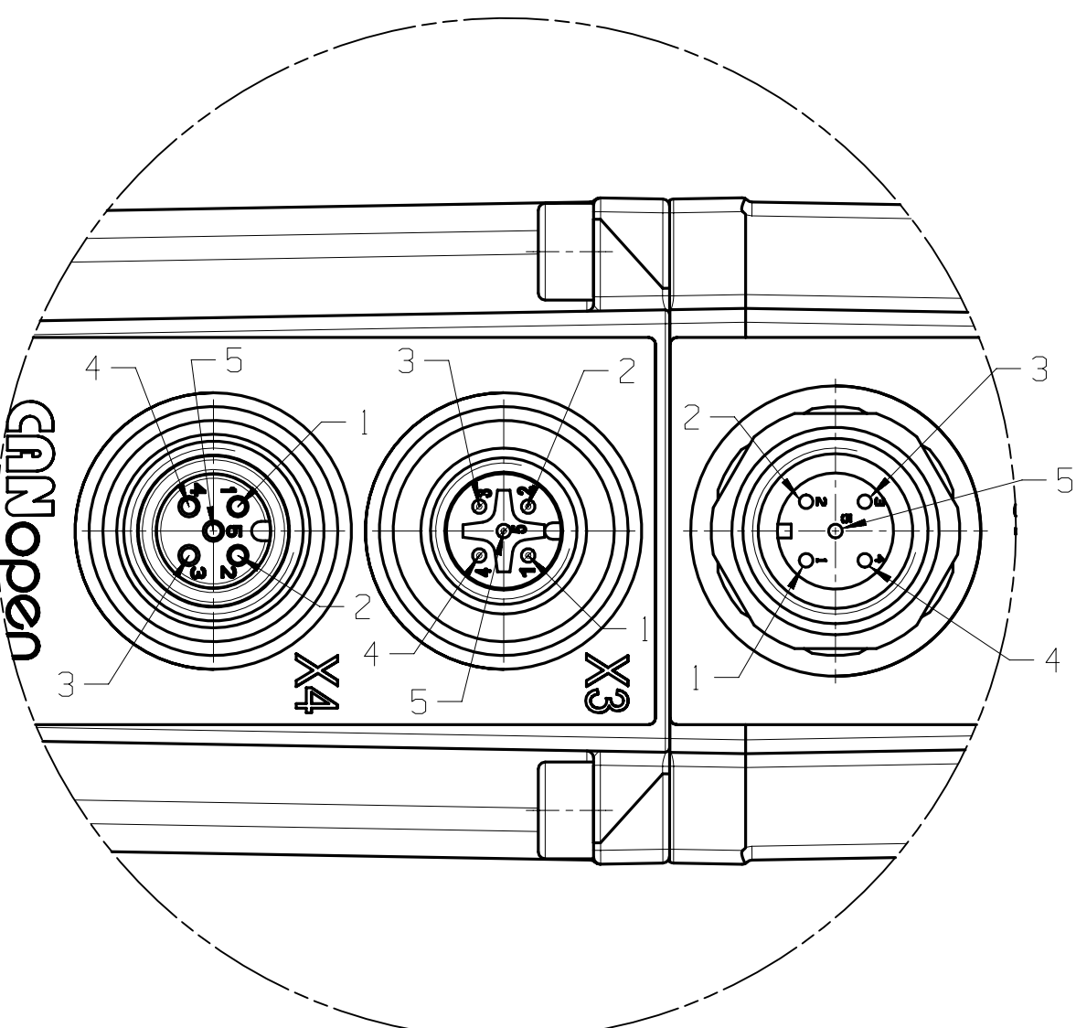
DETAIL B M 2:1
