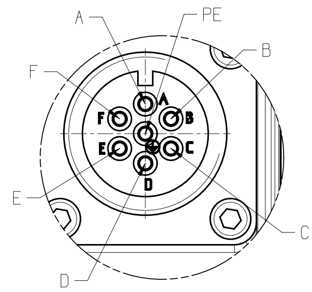
DETAIL A M 2:1
