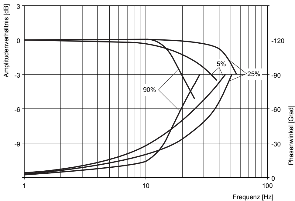
Abb. 94: Frequenzgang für Ventile D945K, standard, Stufenkolben K10
