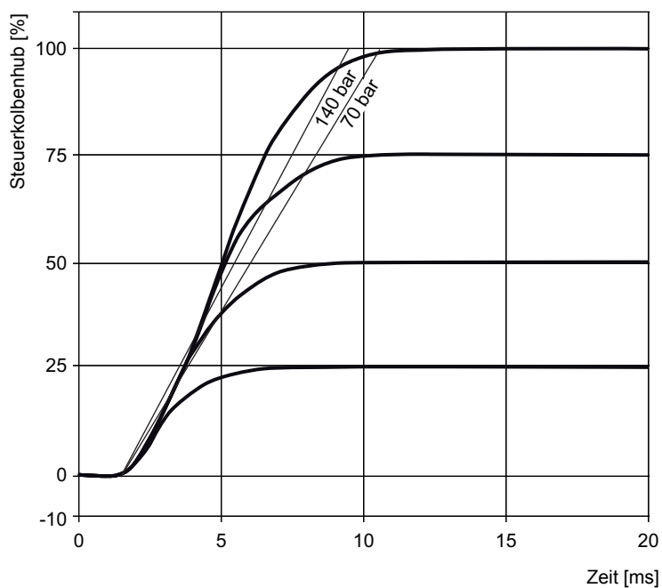
Abb. 60: Sprungantwort für Ventile D941K, standard
