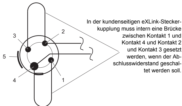
Abb. 46: Anschluss Ventil Profibus mit ventிலinternem Abschlusswiderstand
