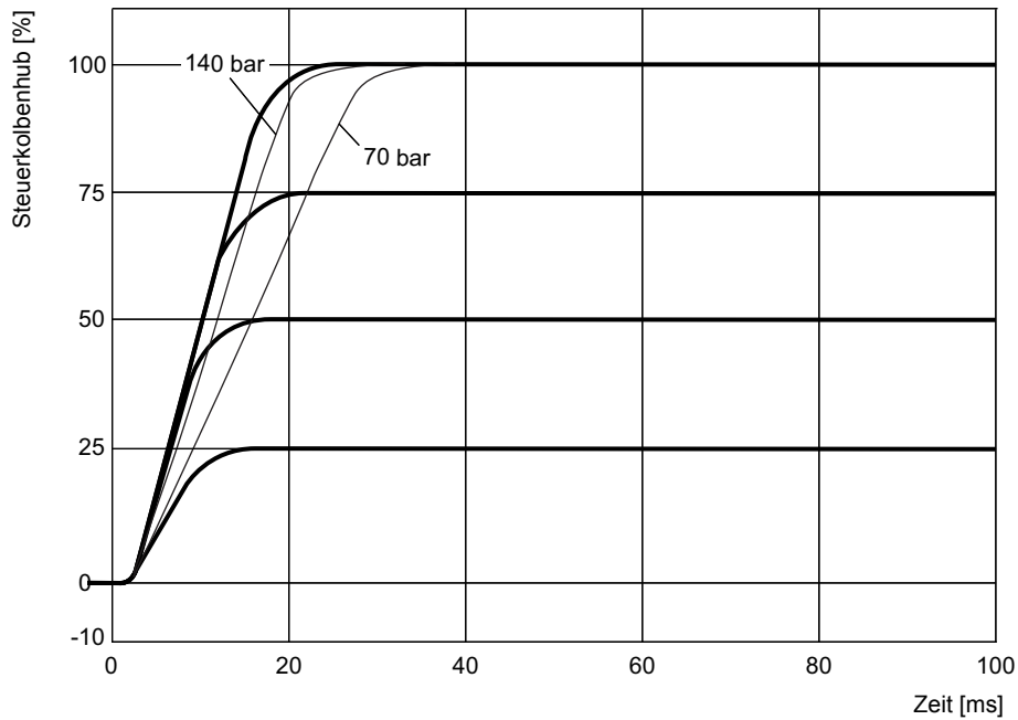
Abb. 97: Sprungantwort für Ventile D945K, standard, Stufenkolben K15
