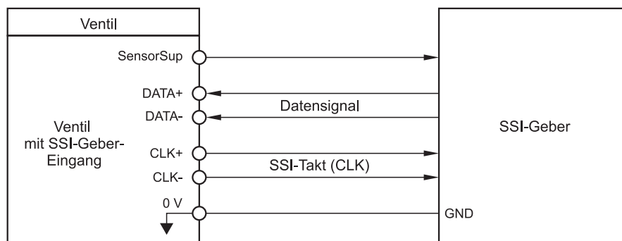
Abb. 40: Anschlussbild mit SSI-Geber
