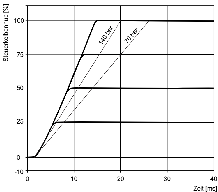
Abb. 76: Sprungantwort für Ventile D943K, standard
