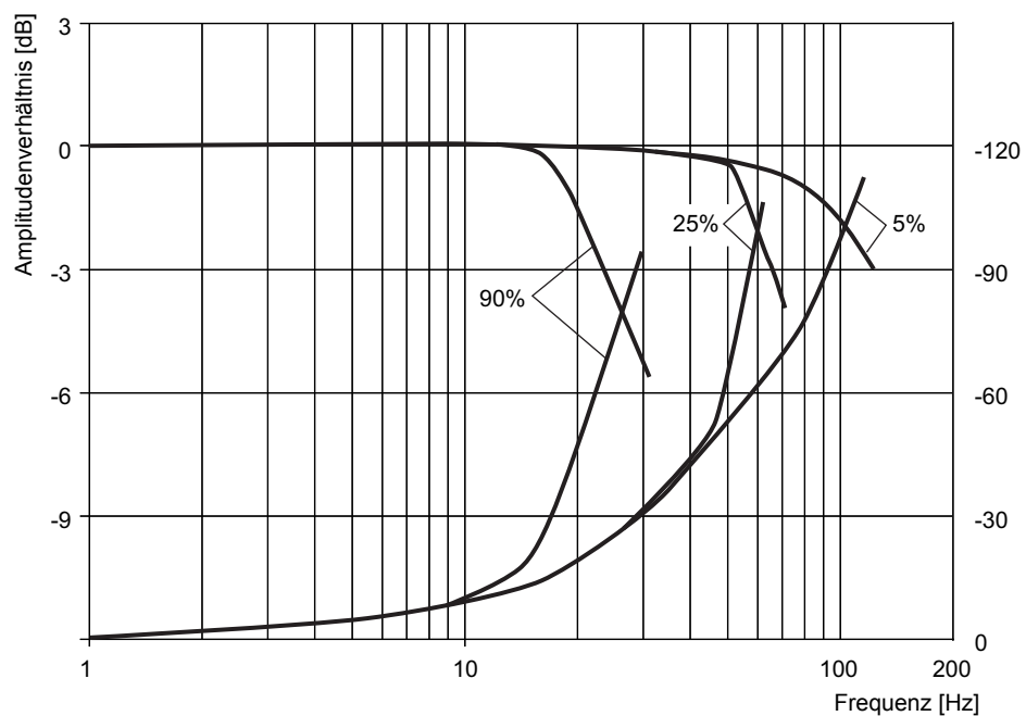
Abb. 85: Frequenzgang für Ventile D944K, standard
