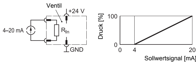
Abb. 13: Differenzieller Druckfunktion-Sollwerteingang 4–20 mA (Schaltung und Kennlinie)
