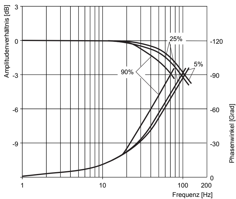
Abb. 61: Frequenzgang für Ventile D941K, standard
