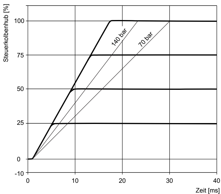
Abb. 78: Sprungantwort für Ventile D943K, vertrimmt
