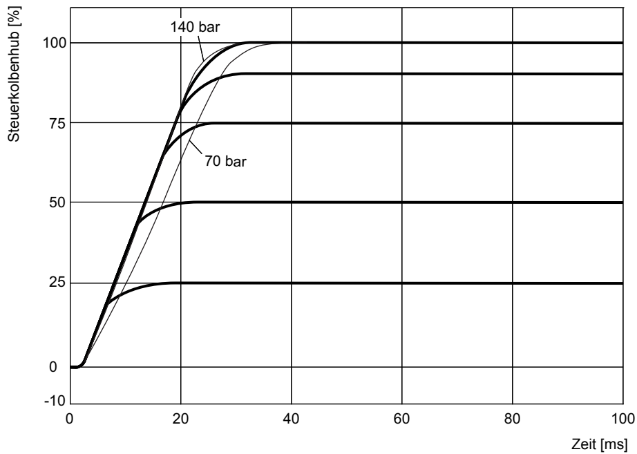
Abb. 95: Sprungantwort für Ventile D945K, vertrimmt, Stufenkolben K10
