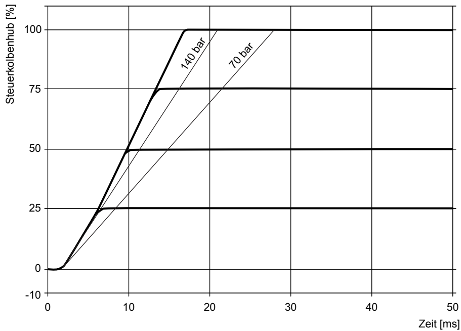
Abb. 84: Sprungantwort für Ventile D944K, standard
