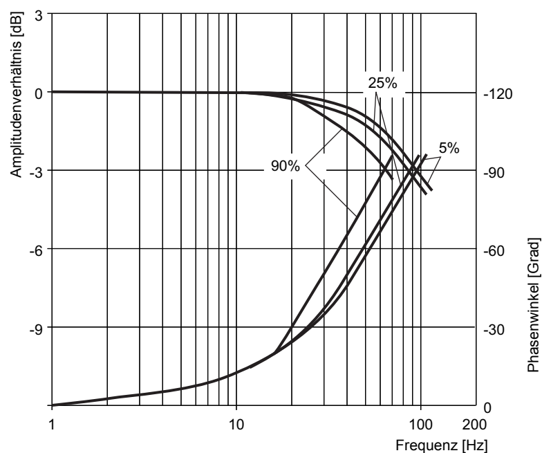
Abb. 63: Frequenzgang für Ventile mit D941K, vertrimmt
