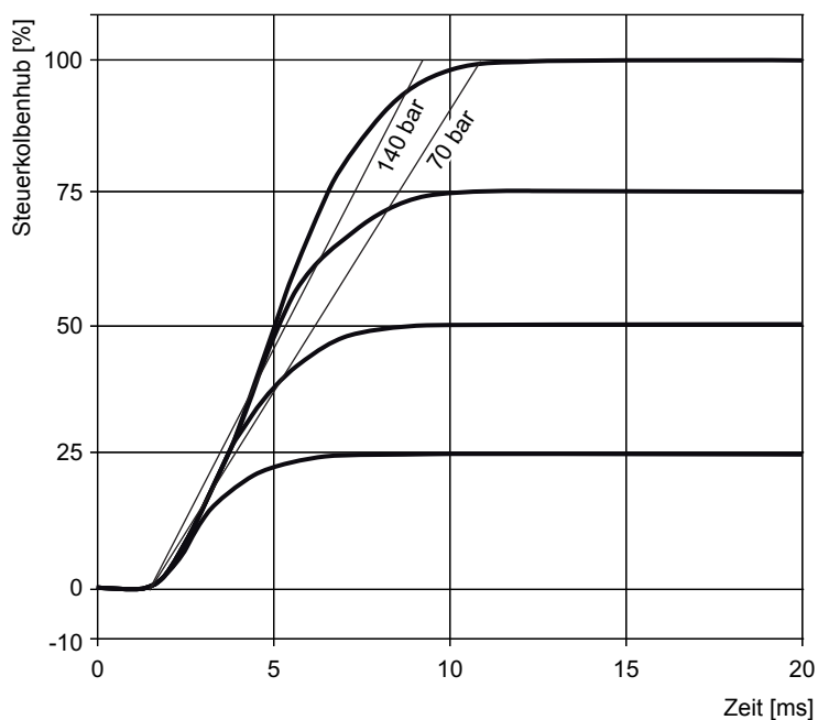
Abb. 62: Sprungantwort für Ventile D941K, vertrimmt
