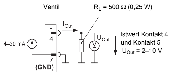
Abb. 39: Schaltung zur Wandlung der Istwertausgangssignale I_{Out}
