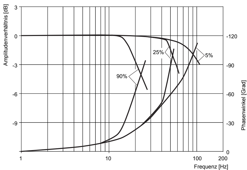
Abb. 87: Frequenzgang für Ventile D944K, vertrimmt
