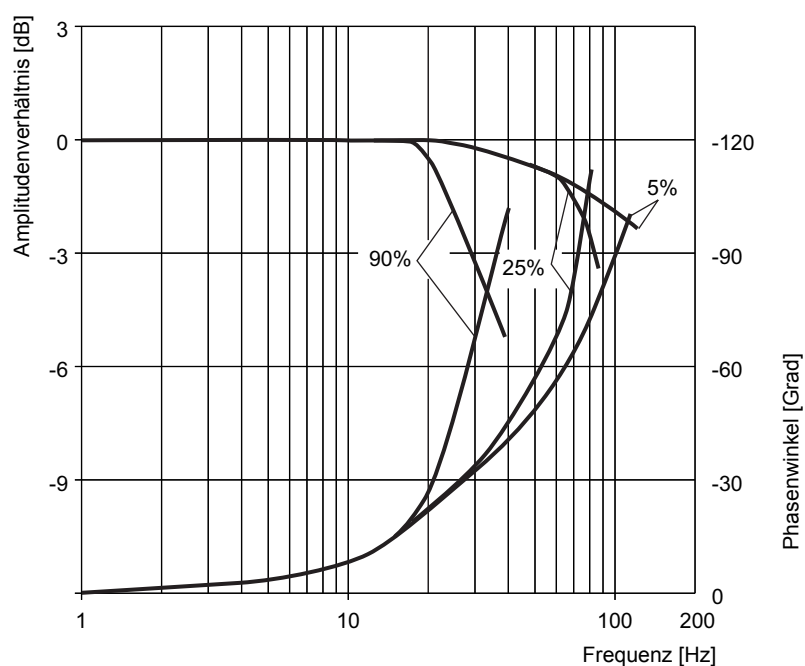
Abb. 71: Frequenzgang für Ventile D942K, vertrimmt
