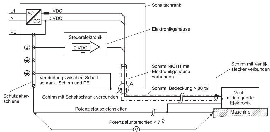
Abb. 32: Potenzialausgleich und Schutzerdung von Maschinen (siehe auch EN 60204-1 ) sowie Schirmung unserer Ventile mit integrierter Elektronik
