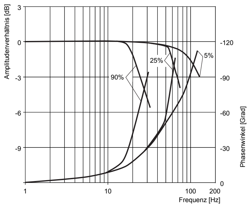
Abb. 77: Frequenzgang für Ventile D943K, standard
