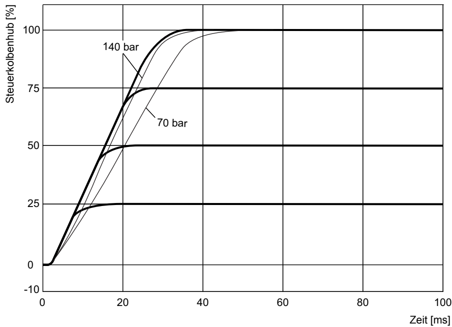
Abb. 99: Sprungantwort für Ventile D945K, vertrimmt, Stufenkolben K15
