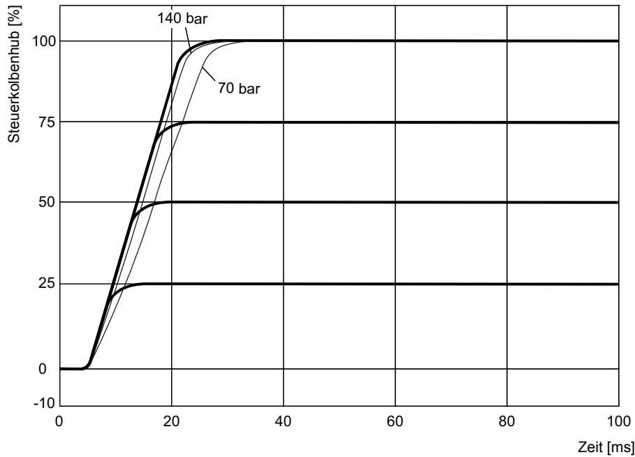
Abb. 93: Sprungantwort für Ventile D945K, standard, Stufenkolben K10
