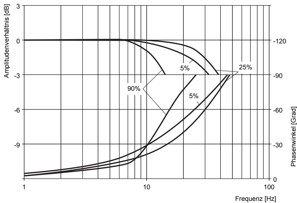
Abb. 96: Frequenzgang für Ventile D945K, vertrimmt, Stufenkolben K10
