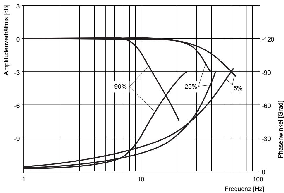
Abb. 100: Frequenzgang für Ventile D945K, vertrimmt, Stufenkolben K15
