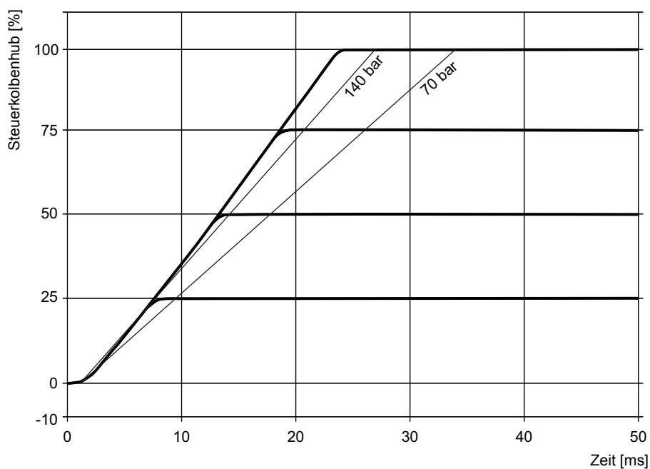
Abb. 86: Sprungantwort für Ventile D944K, vertrimmt
