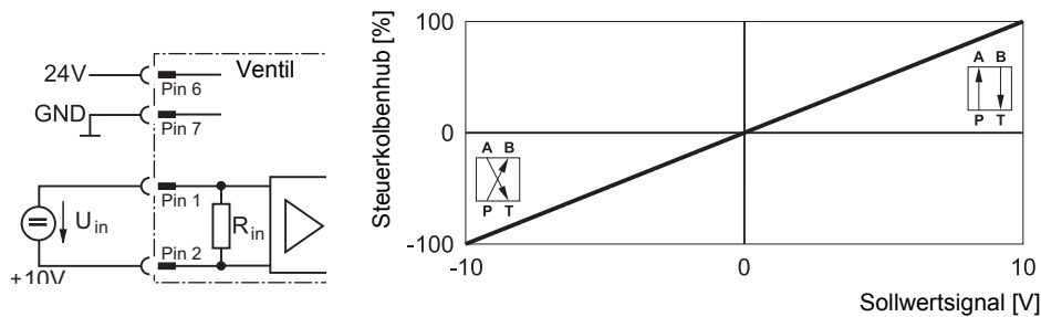
Abb. 8: Potenzialfreier Volumenstromfunktion-Sollwerteingang \pm 10 V (Schaltung und Kennlinie)
