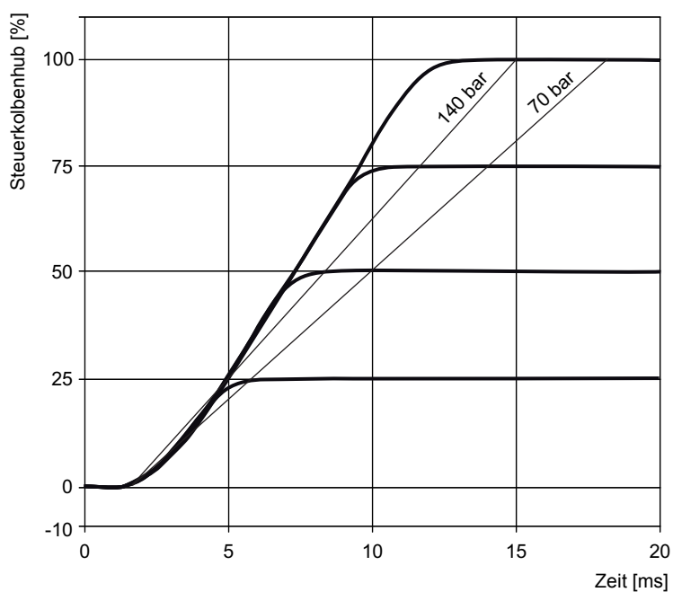
Abb. 70: Sprungantwort für Ventile D942K, vertrimmt
