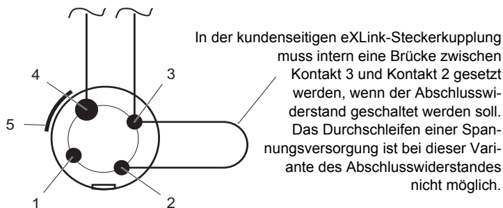
Abb. 43: Anschluss Ventil CAN-Bus mit ventilinternem Abschlusswiderstand
