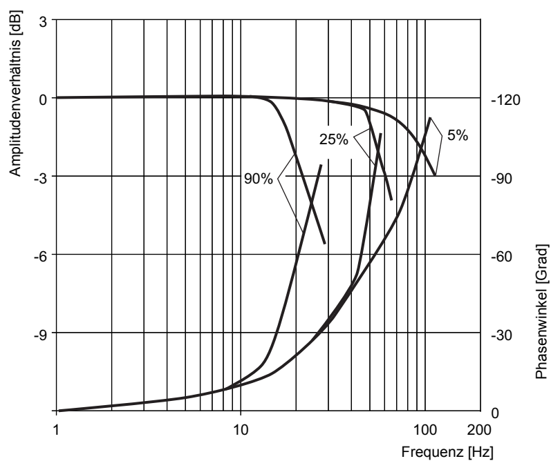
Abb. 79: Frequenzgang für Ventile mit D943K, vertrimmt
