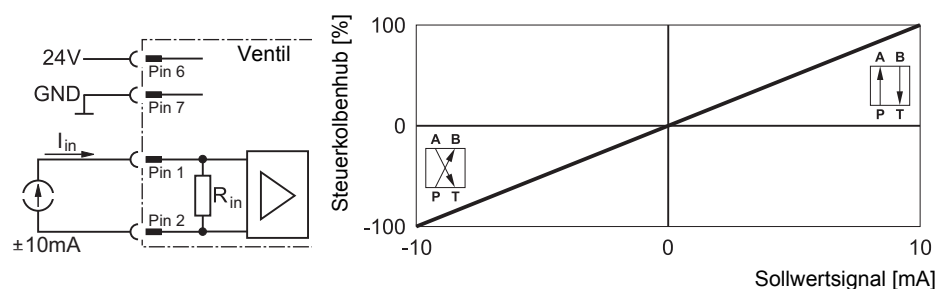
Abb. 9: Potenzialfreier Volumenstromfunktion-Sollwerteingang \pm 10 mA (Schaltung und Kennlinie)
