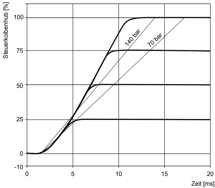
Abb. 68: Sprungantwort für Ventile D942K, standard
