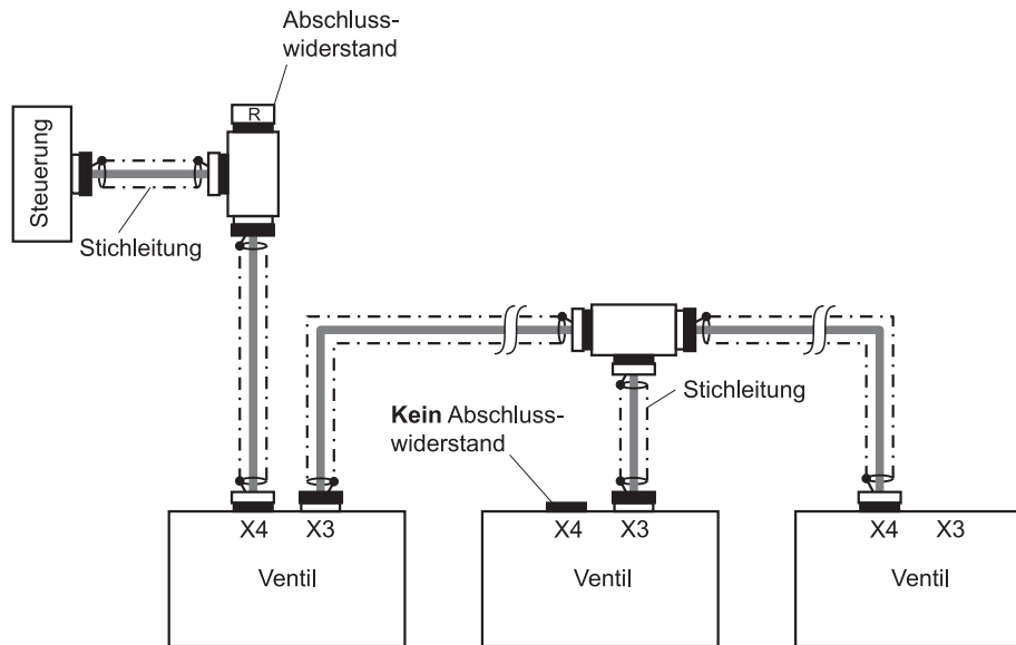
Abb. 45: Profibus-DP-Verdrahtungsschema
