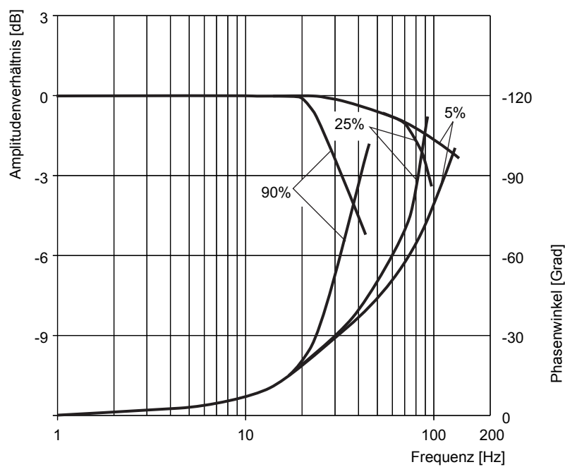
Abb. 69: Frequenzgang für Ventile D942K, standard
