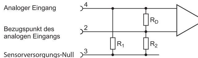
Abb. 41: Ersatzschaltbild des analogen Eingangs
