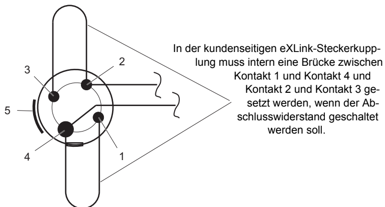
Abb. 58: Anschluss Ventil Profibus mit Abschlusswiderstand
