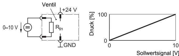
Abb. 14: Differenzieller Druckfunktion-Sollwerteingang 0–10 V (Schaltung und Kennlinie)
