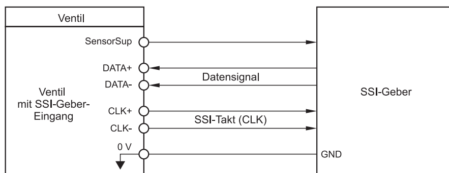
Abb. 52: Anschlussbild mit SSI-Geber
