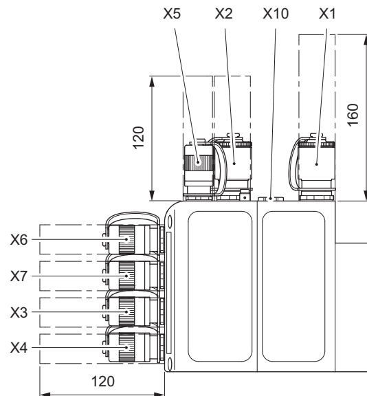
Abb. 33: Anordnung der Anbaustecker am Gehäuse der Ventilelektronik (Maximalausstattung)
