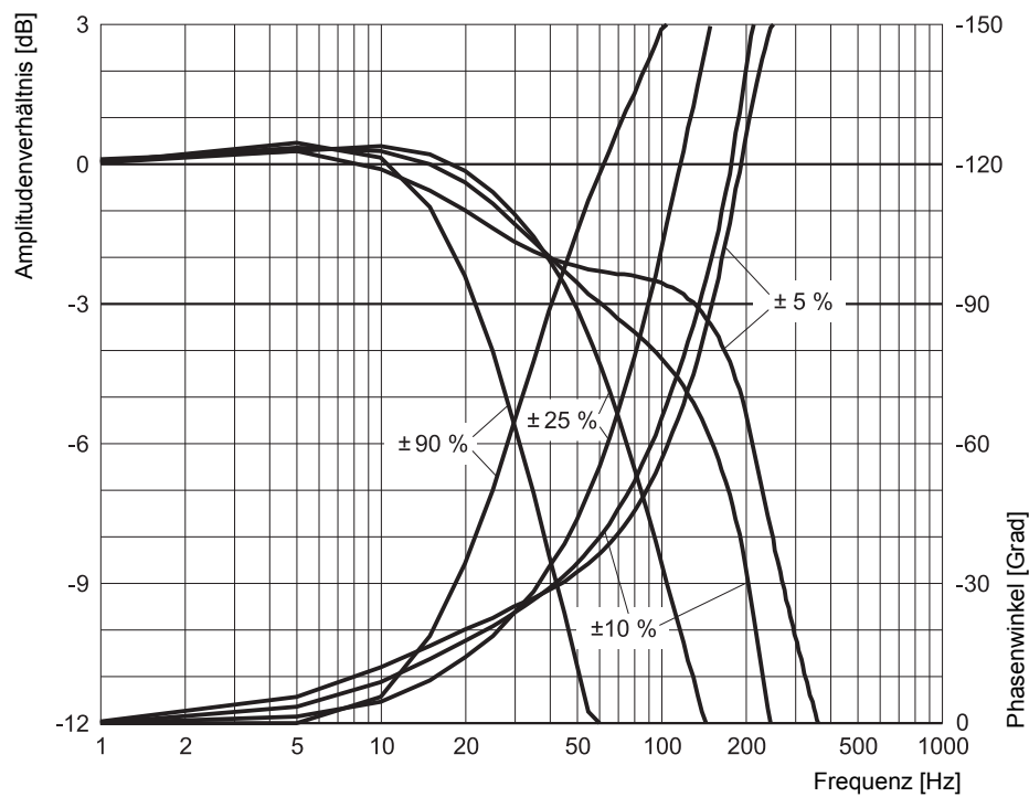
Abb. 29: Frequenzgang des Steuerkolbenhubs für Ventile mit Q_N = 100 \text{ l/min}
