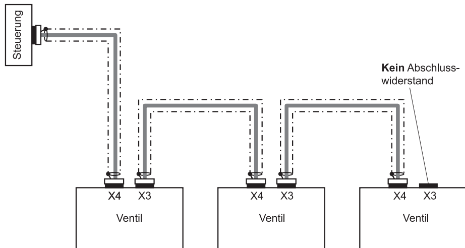
Abb. 59: EtherCAT-Verdrahtungsschema
