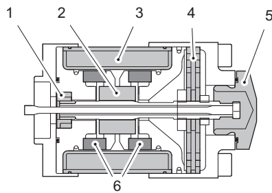
Abb. 2: Prinzipdarstellung eines Permanentmagnet-Linearmotors
