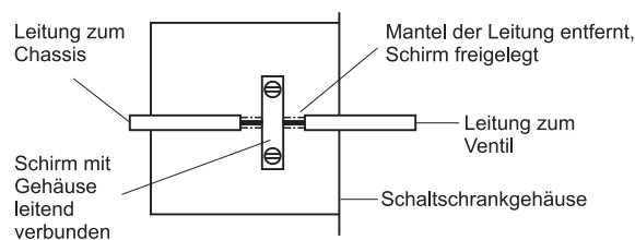
Abb. 44: Anschluss des Schirms am Schaltschrankgehäuse (Einzelheit A zu Abb. 43)
