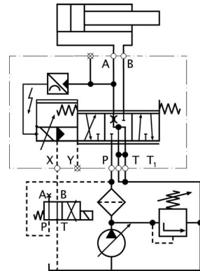
Wahlweise Y extern
